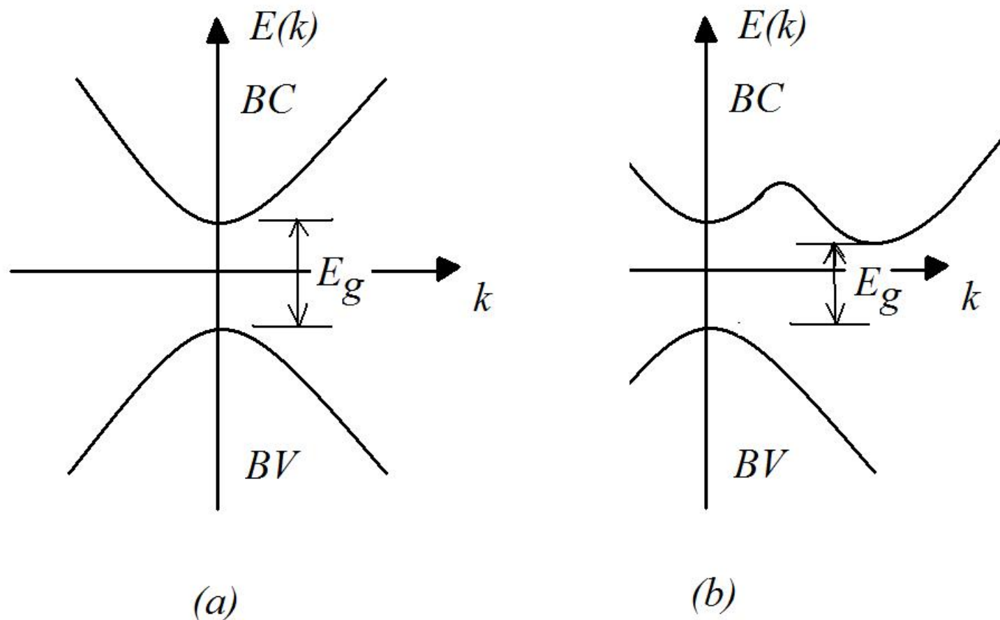
Figure 1: (a) Gap Direto e (b) Gap Indireto.
