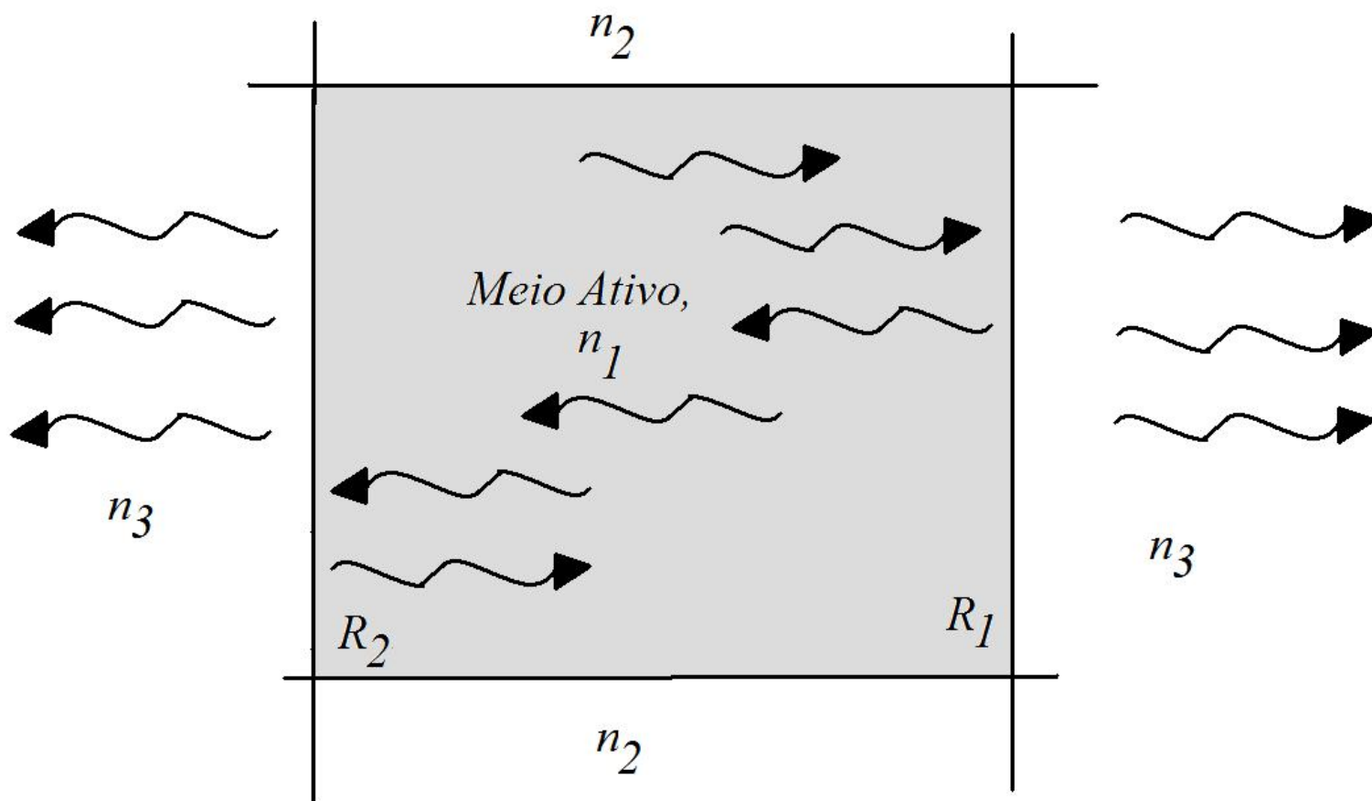
Figure 4: Estrutura típica de um Laser. O meio ativo n_1 é delimitado por duas interfaces de refletividades R_1 e R_2 .
