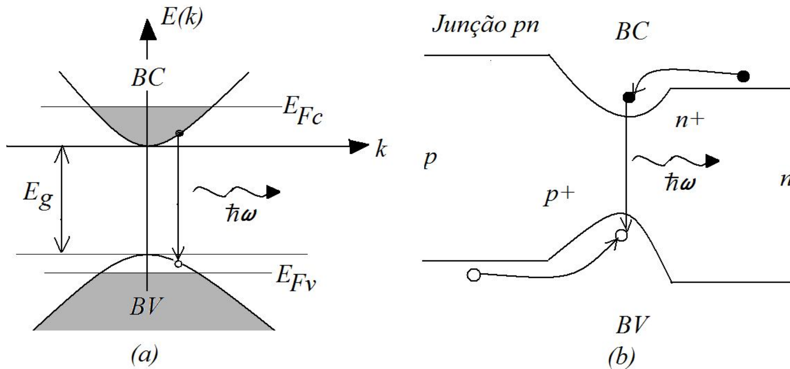
Figure 5: (a) Estrutura de Bandas com Gap Direto: processo de recombinação radiativa. (b) Junção pn típica: as regiões altamente dopadas p^+ e n^+ permitem a formação da estrutura de bandas mostrada em (a) na região de transição, fazendo uma armadilha para os portadores que se recombinam, emitindo fótons.
