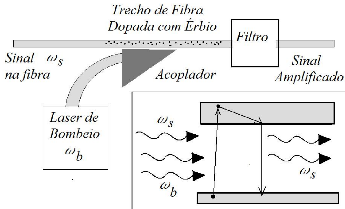
Figure 7: Esquema Típico de um EDFA. Geralmente \lambda_b = 1.48\mu\text{m} e \lambda_s = 1.55\mu\text{m} .
