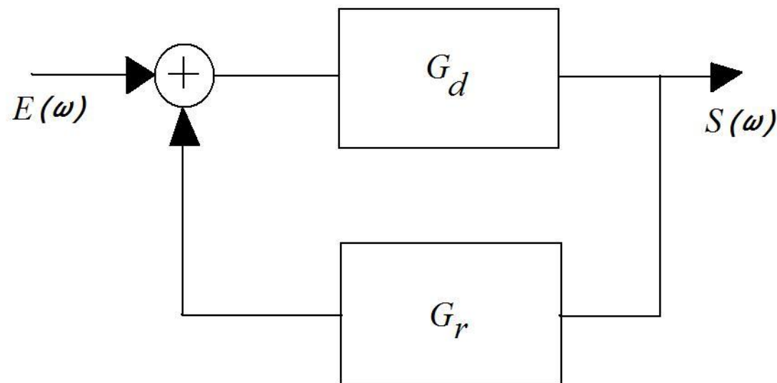
Figure 3: Sistema com realimentação
