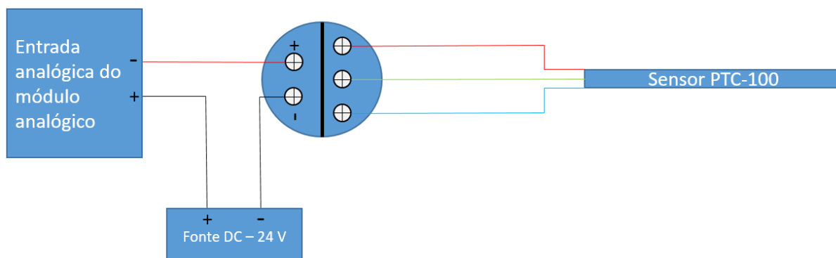
FIGURA 18 - ESQUEMÁTICO DE CONEXÃO
