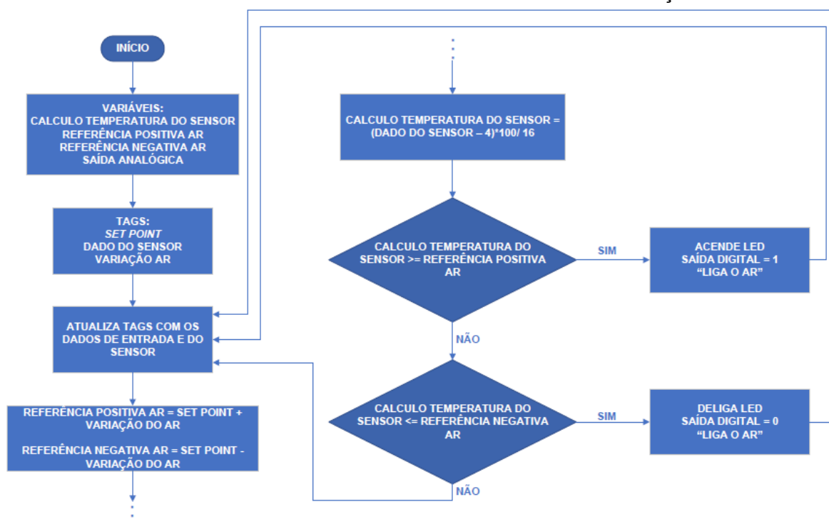
FIGURA 24 - FLUXOGRAMA DA LÓGICA DE PROGRAMAÇÃO
