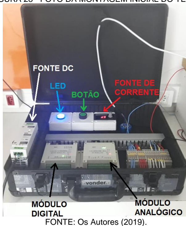
FIGURA 28 - FOTO DA MONTAGEM INICIAL DO TESTE
