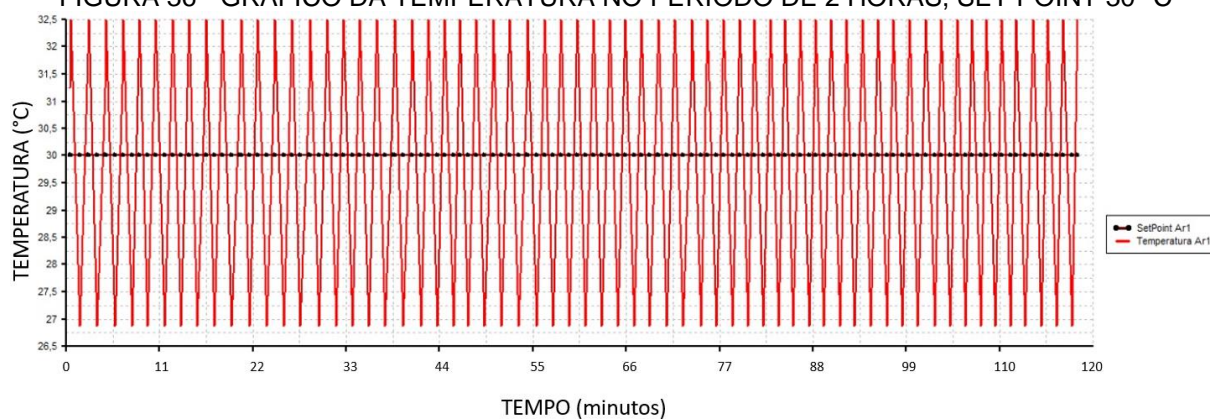
FIGURA 36 - GRÁFICO DA TEMPERATURA NO PERÍODO DE 2 HORAS, SET POINT 30 °C
