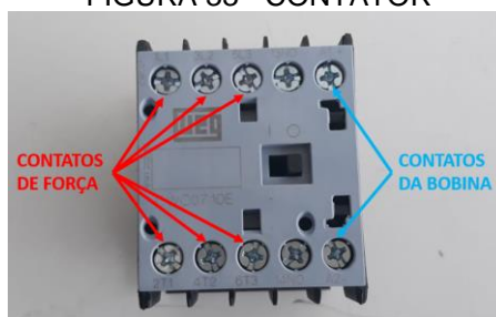
FIGURA 33 - CONTATOR
