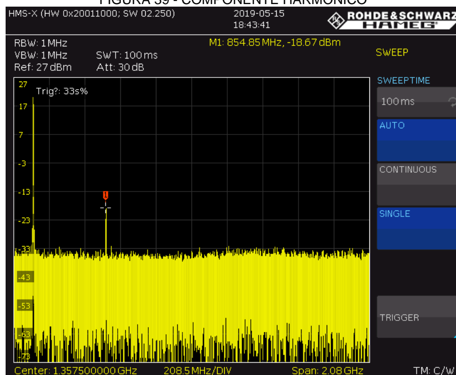
FIGURA 39 - COMPONENTE HARMÔNICO
