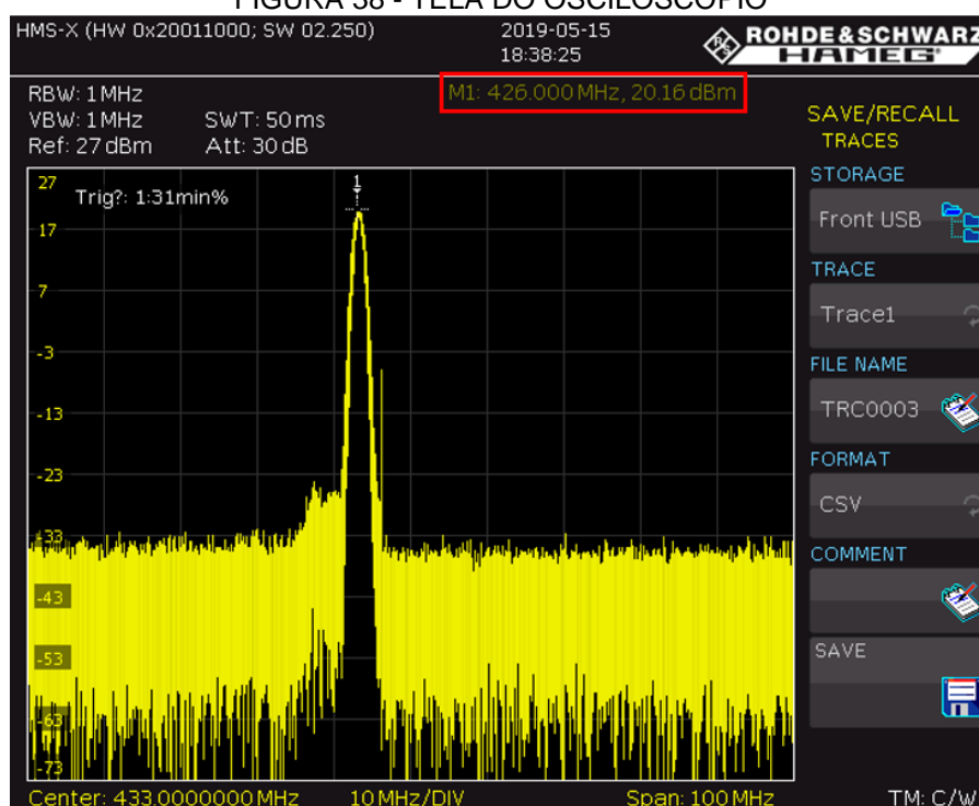
FIGURA 38 - TELA DO OSCILOSCÓPIO
