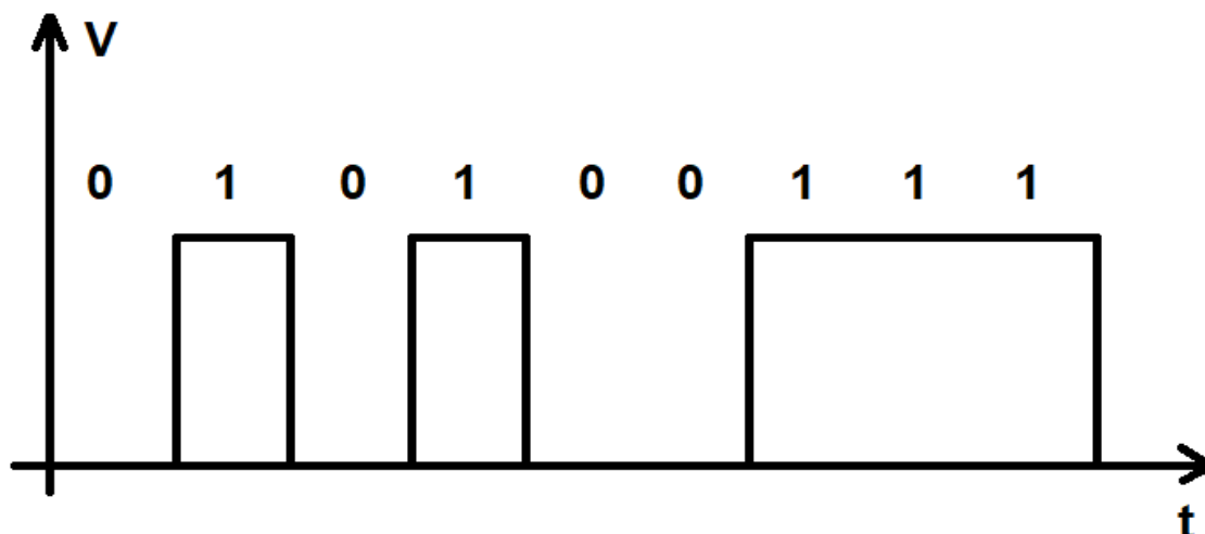
FIGURA 4 - EXEMPLO DE SINAL DIGITAL
