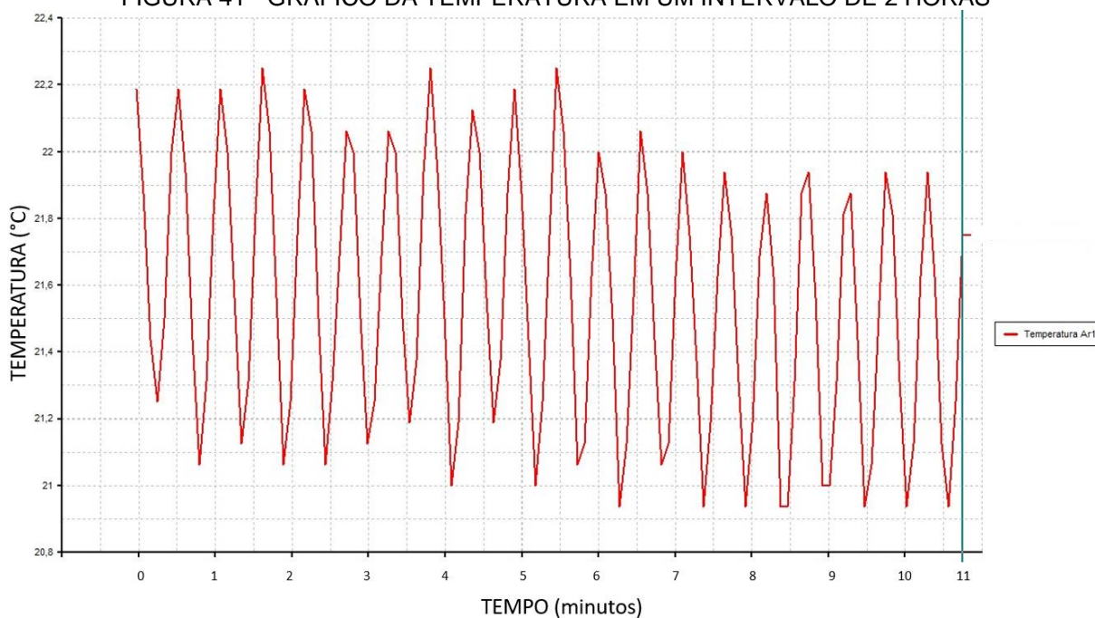
FIGURA 41 - GRÁFICO DA TEMPERATURA EM UM INTERVALO DE 2 HORAS
