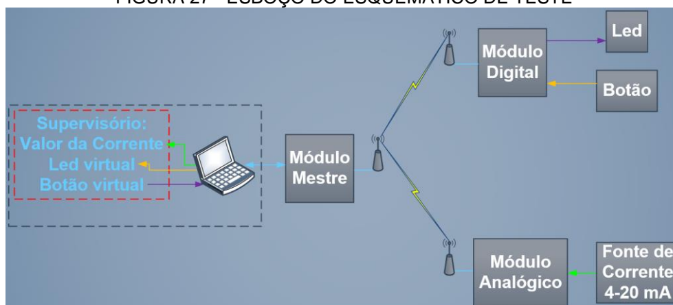
FIGURA 27 - ESBOÇO DO ESQUEMÁTICO DE TESTE
