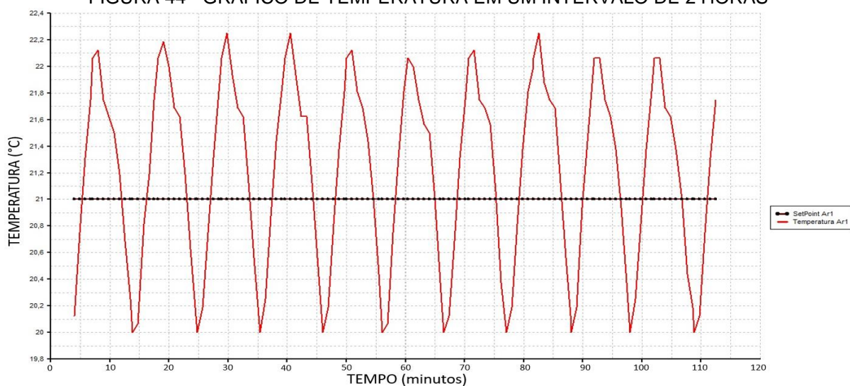
FIGURA 44 - GRÁFICO DE TEMPERATURA EM UM INTERVALO DE 2 HORAS
