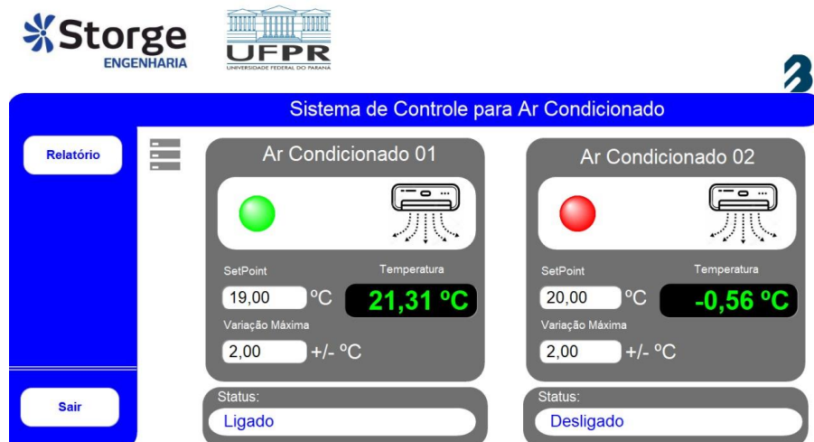
FIGURA 25 - IMAGEM DO SISTEMA SUPERVISÓRIO
