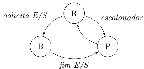
Figure 1: Diagrama de estados possíveis para processos
