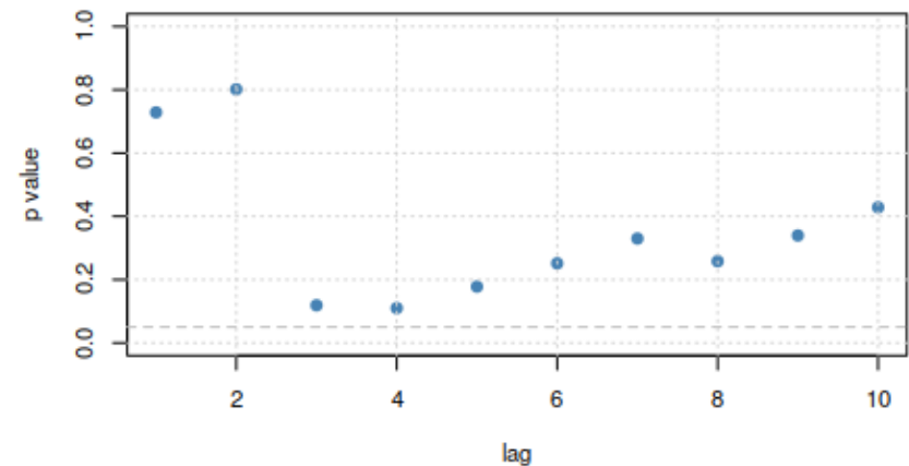
Ljung-Box p-values
