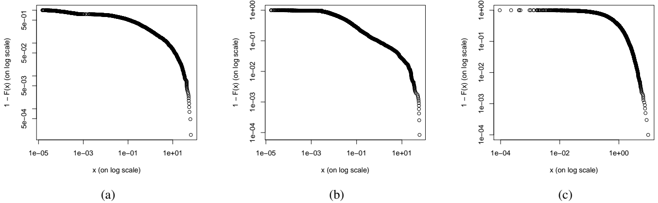
Fig. 3. Gráfico da LLCD para: (a) primeira amostra (b) segunda amostra e (c) distribuição exponencial
