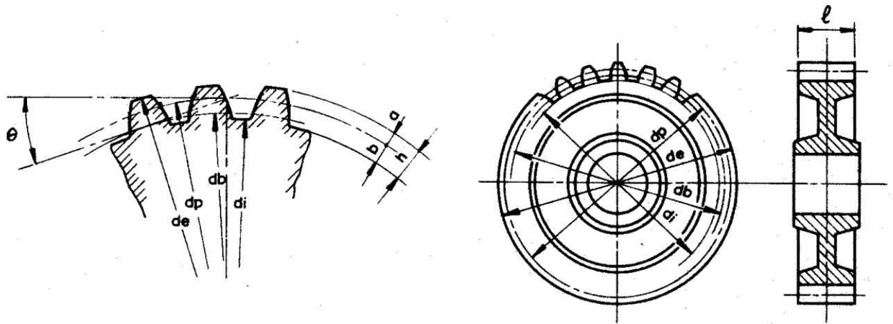
Figura 6 – Parâmetros da engrenagem.
