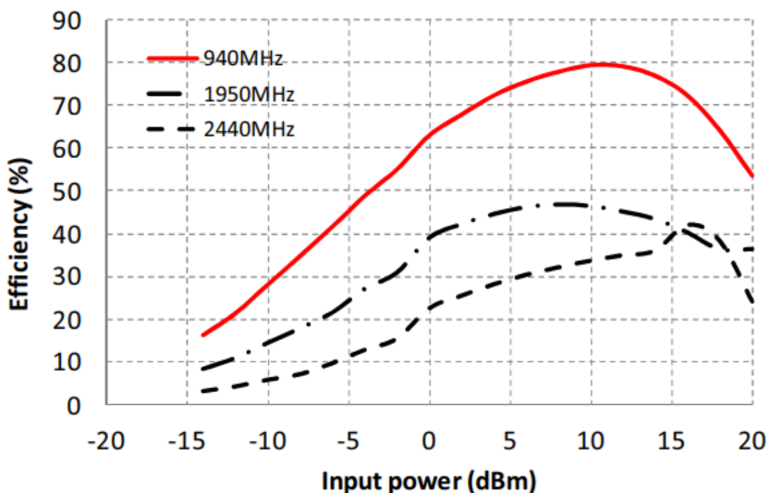
Figura 9 - Eficiência medida do retificador [21].
