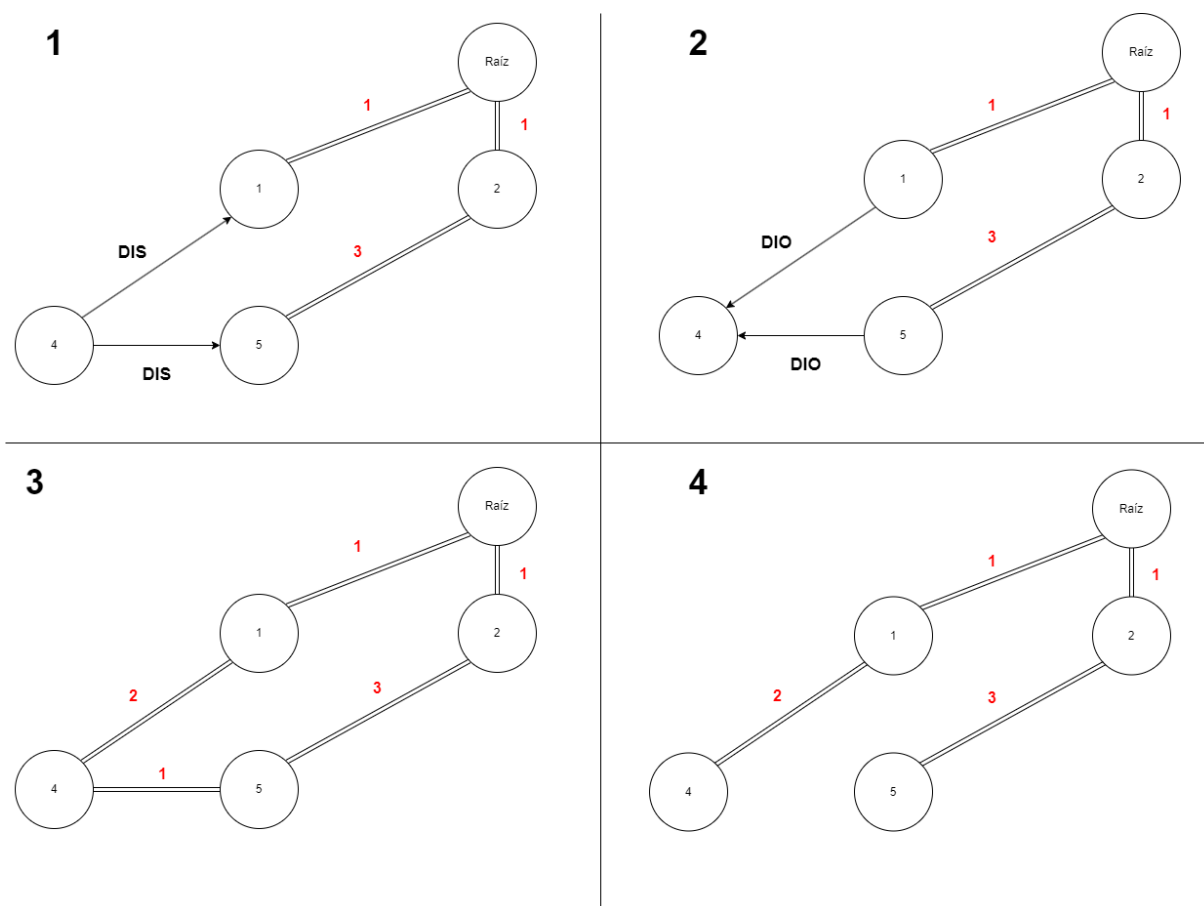
Figura 6 - Ilustração do funcionamento das mensagens DIS e DIO.
