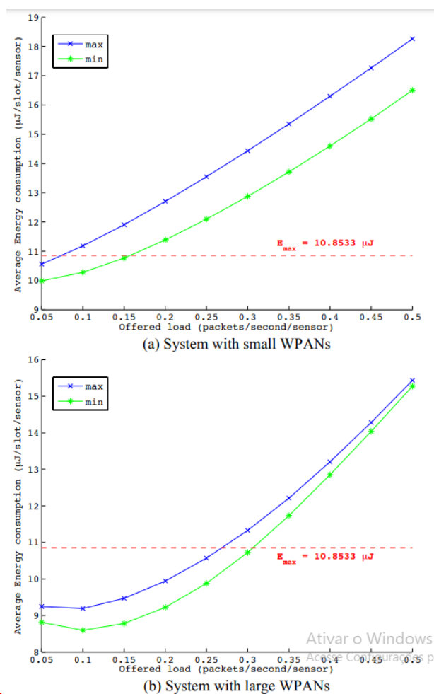
Figura 3 - Consumo médio de energia em função da frequência de envio de pacotes por sensor em grandes e pequenas WPANs [18].
