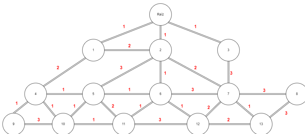
Figura 5 - Alcance dos nós da rede com o protocolo RPL e retransmissões necessárias.
