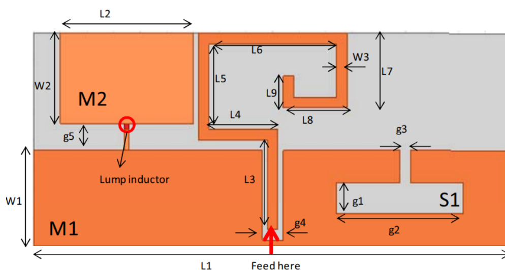
Figura 8 - Design da antena de três bandas.
