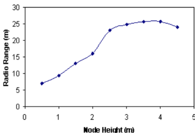
Figura 4 - Alcance de rádios Bluetooth e IEEE 802.11 na faixa de 2,4 GHz em função da altura da antena em plantações agrícolas [16].
