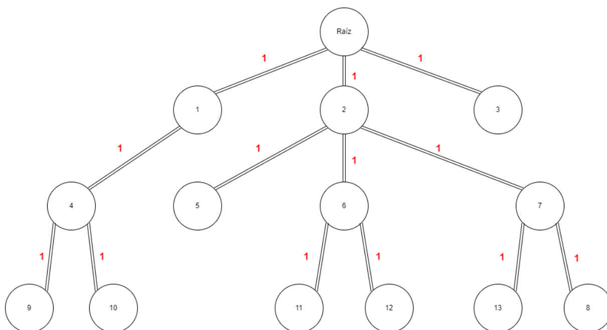
Figura 7 - Topologia da rede com o protocolo RPL usando a OF0.
