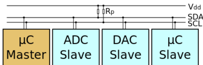
FIGURA 2.2 – Exemplo de comunicação I2C
