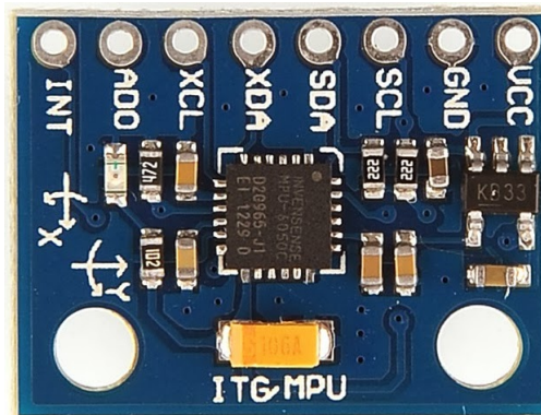
FIGURA 3.2 – Placa do módulo MPU-6050
