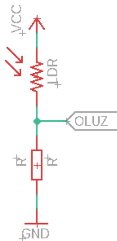
FIGURA 6 - DIVISOR DE TENSÃO DO LDR
