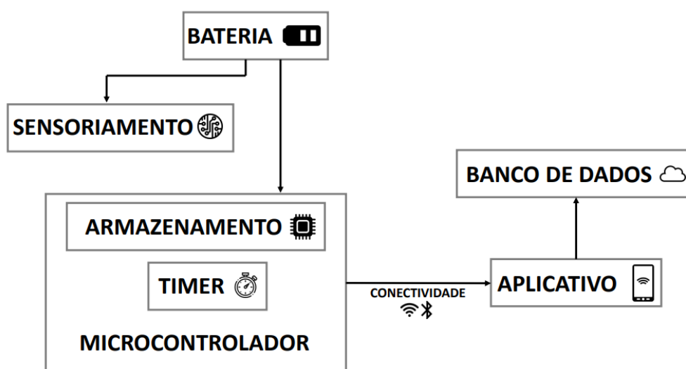
FIGURA 5 - DIAGRAMA DE BLOCOS DO PROJETO
