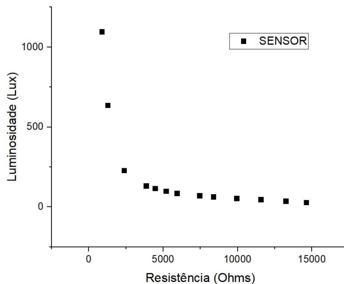
FIGURA 11 - CARACTERIZAÇÃO DO SENSOR LDR
