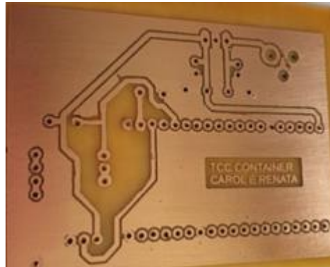
FIGURA 18 - PCB CONFECCIONADA
