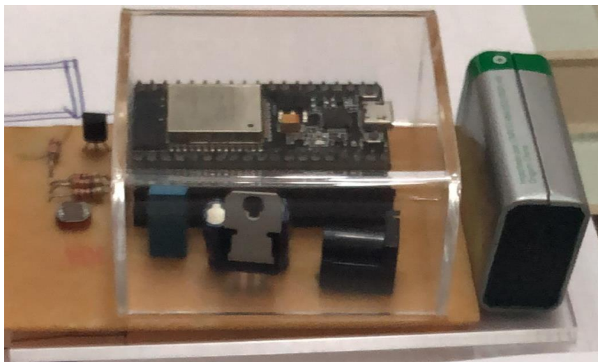
FIGURA 19 - PROTÓTIPO COM ENCAPSULAMENTO ACRÍLICO
