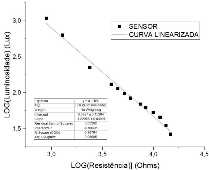
FIGURA 12 - CALIBRAÇÃO DO SENSOR LDR LINEARIZADO
