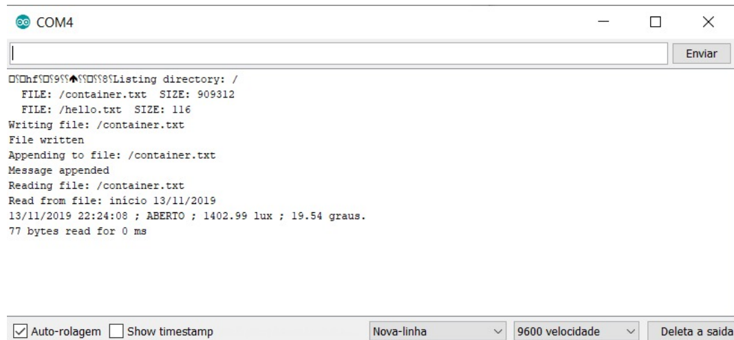
FIGURA 8 - PORTA SERIAL COM TAMANHO DO VETOR ARMAZENADO
