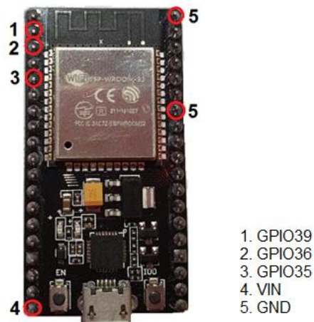
FIGURA 13 - ESP32 E PORTAS UTILIZADAS
