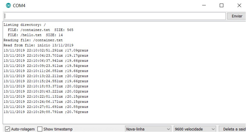
FIGURA 25 - PORTA SERIAL COM RESULTADO PARCIAL
