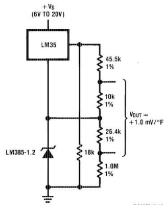
FIGURE 10. Fahrenheit Thermometer
