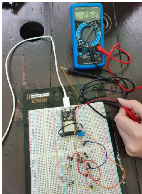
FIGURA 14 - MEDIÇÃO DA CORRENTE DO CIRCUITO
